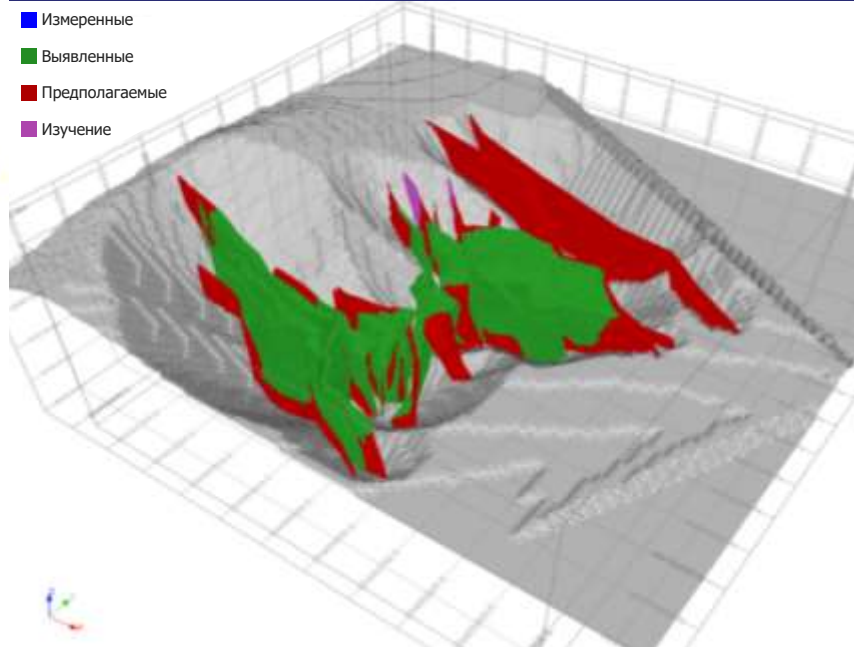
Блочная модель JORC
